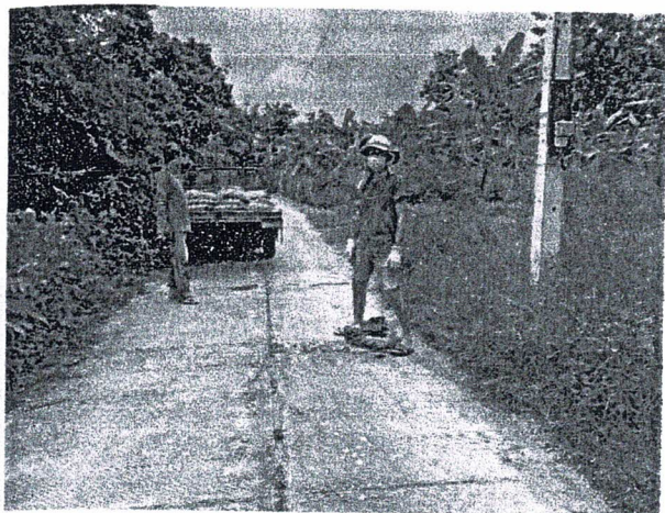
รูปภาพขณะดำเนินการซ่อมแซมถนนคอนกรีตเสริมเหล็กภายในหมู่บ้าน หมู่ที่ 1 บ้านหนองจันทน์
